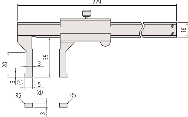
Inside groove type: 536-145
