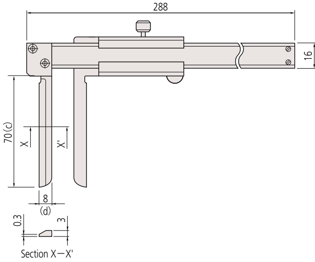
Inside groove type: 536-145
